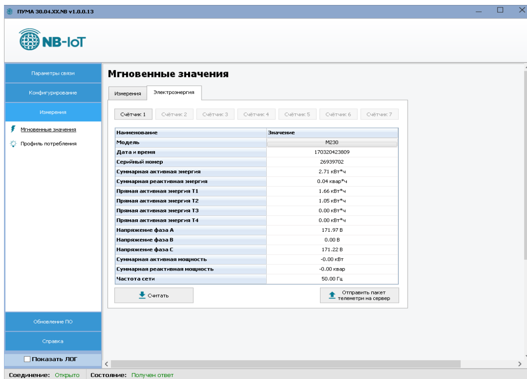
Рис. 19 – Подменю «Мгновенные значения → Электроэнергия»
