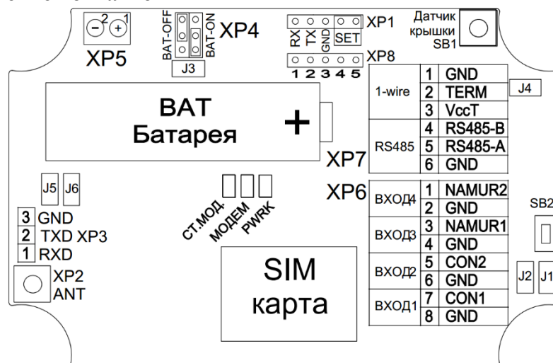
Рис. 2 – Контакты устройства
