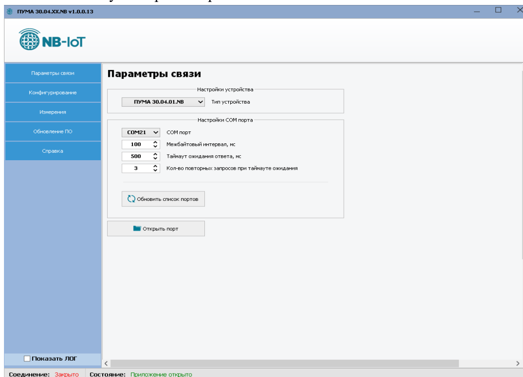
Рис. 7 – Вкладка «Параметры связи»
