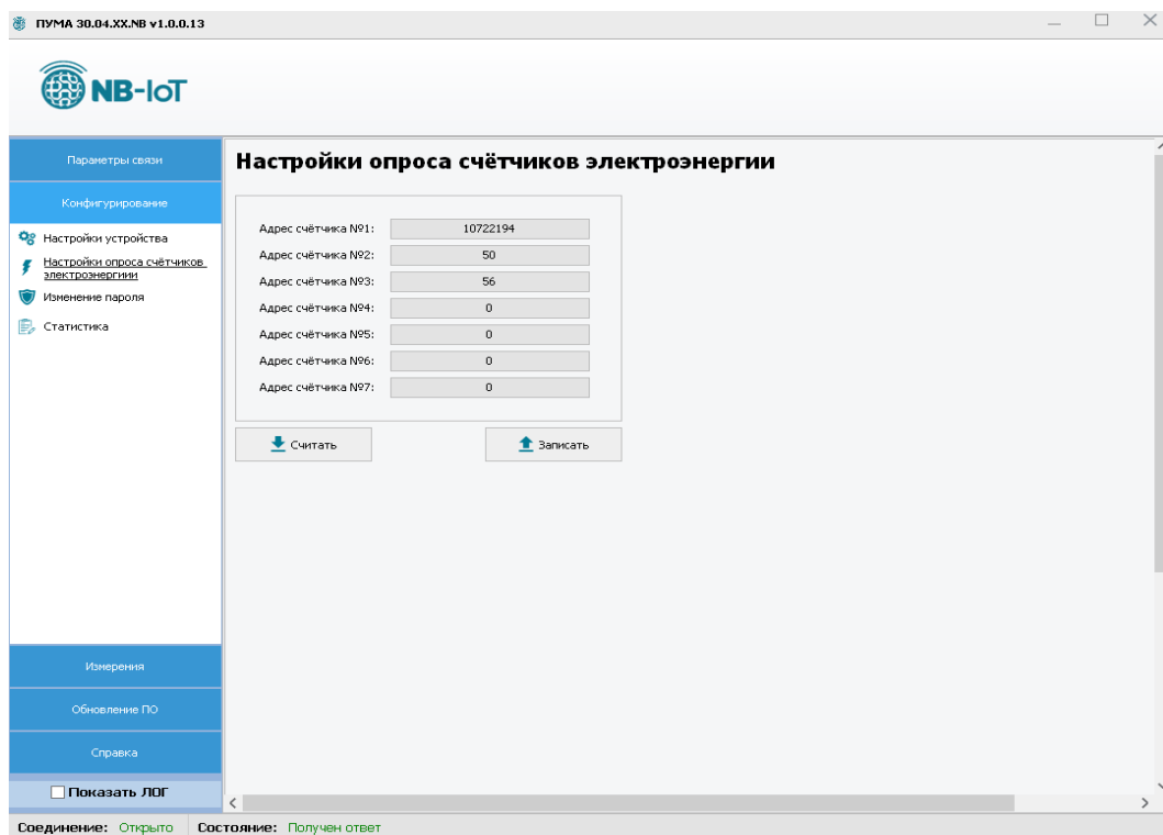
Рис. 15 — Настройка адресов счетчиков
