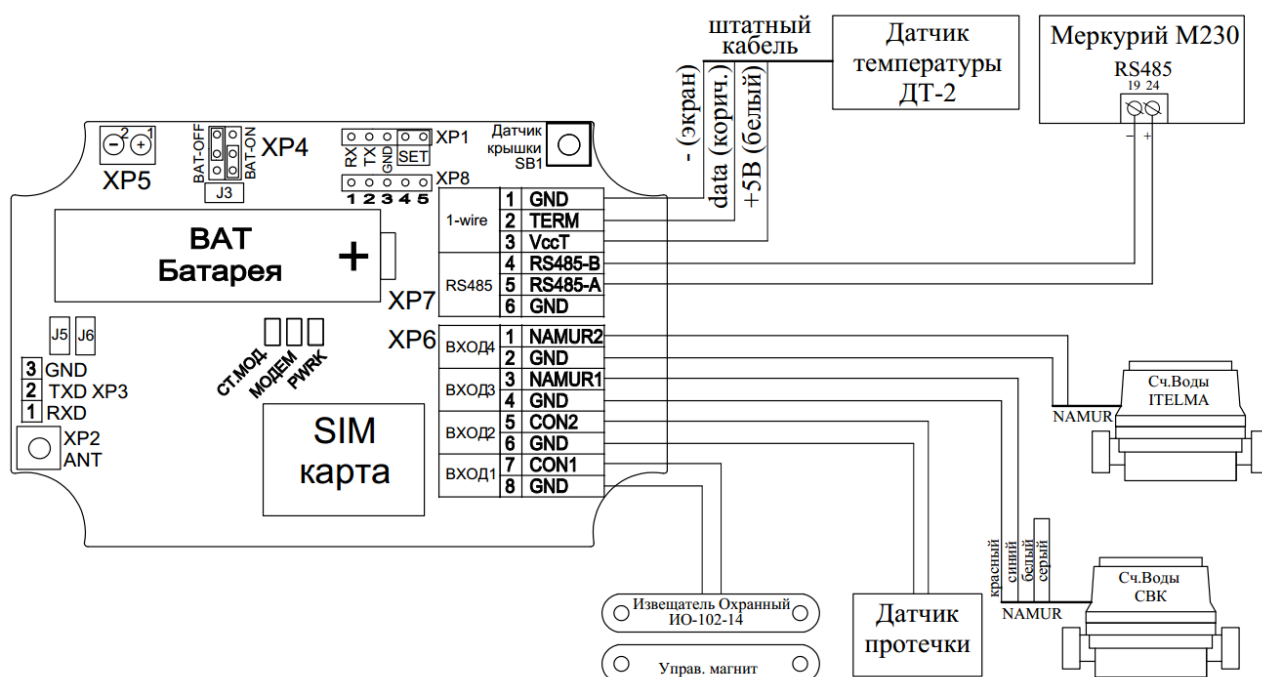
Рис. 3 - Типовая схема подключения устройства
